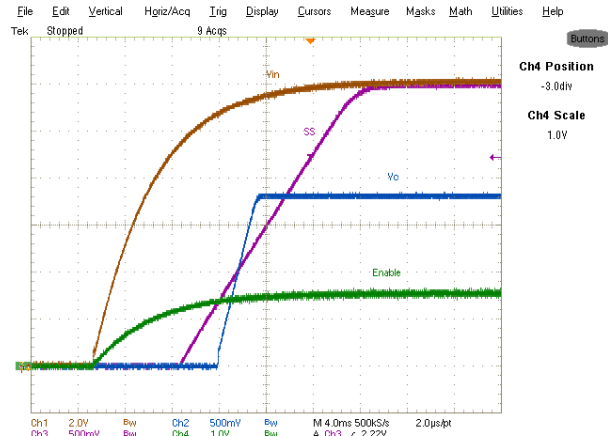
Fig. 17. Start up at 4A Load Ch 1 : V_{in} , Ch 2 : V_o , Ch 3 : V_{ss} , Ch 4 :Enable
