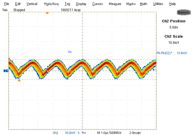
Fig. 20. Output Voltage Ripple, 4A load Ch 2 : V_o
